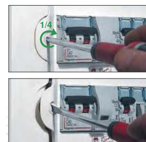
8 POKRIVNE PLOČE Vijci sa 1/4 okreta za brzo i lako skidanje pokrivne ploče (patentirani Legrand sistem). Pokrivne ploče mogu se pojedinačno ukloniti za svaki red (od 2-rednog razdjelnika naviše)
