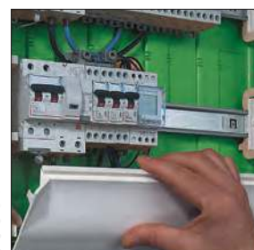
7 JEDNOSTAVAN PRISTUP REDNIM STEZALJKAMA Šasija s pomičnim i zakretnim donjim i gornjim dijelovima omogućuje lakši pristup rednim stezaljkama
