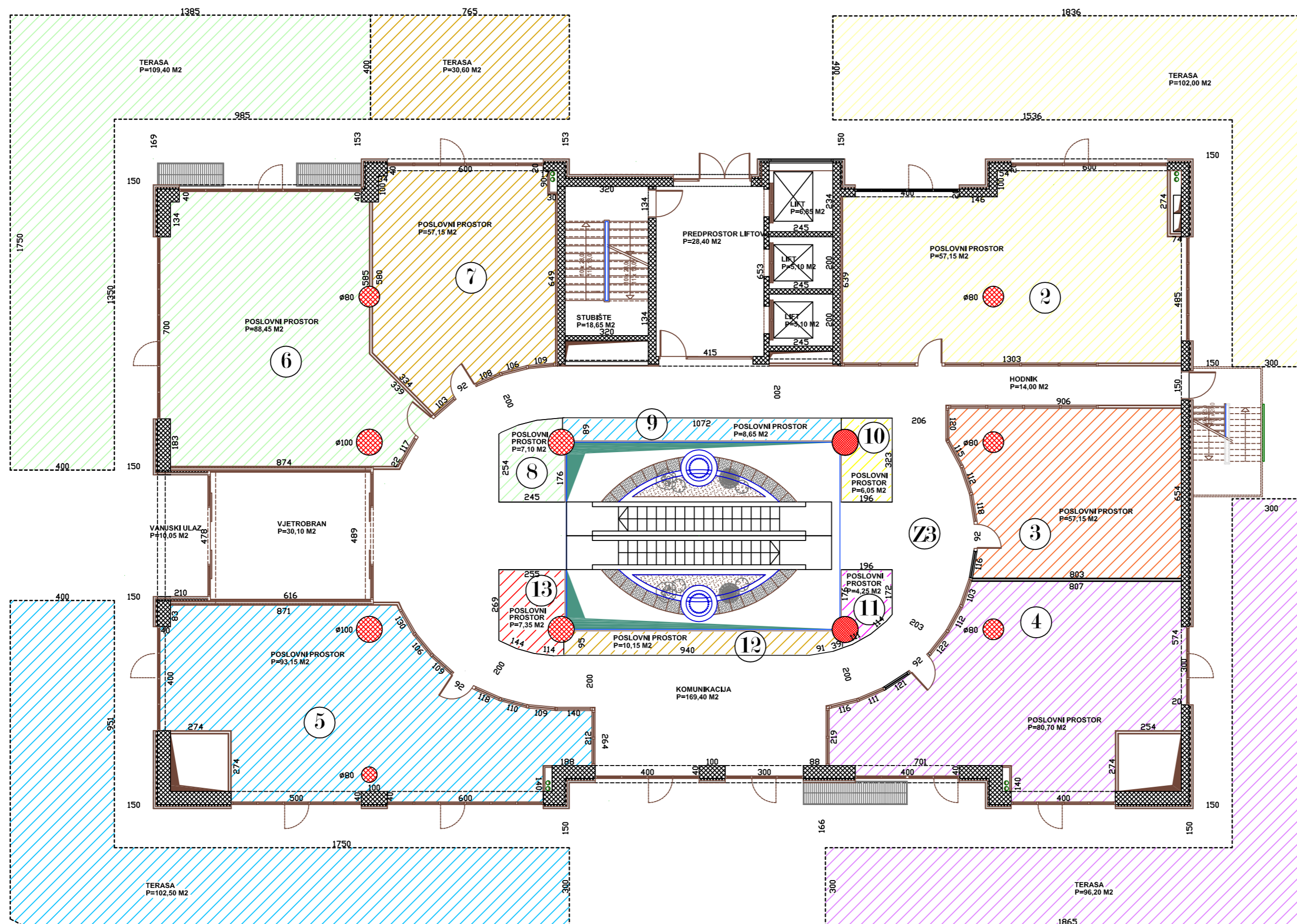
TLOCRT PRIZEMLJA M 1:100
